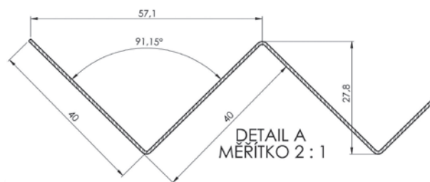
1. Rozvín PL 0,75x1120x2530
